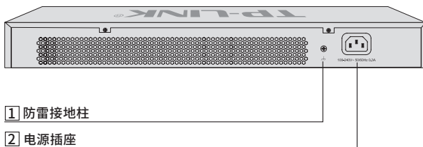
图1-12 TL-SG2226后面板示意图
